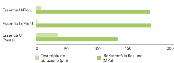
Rezistență la flexiune & testul triplu de abraziune a celor trei vâscozități Essentia Universal shade (Sursa: date GCC R&D)
